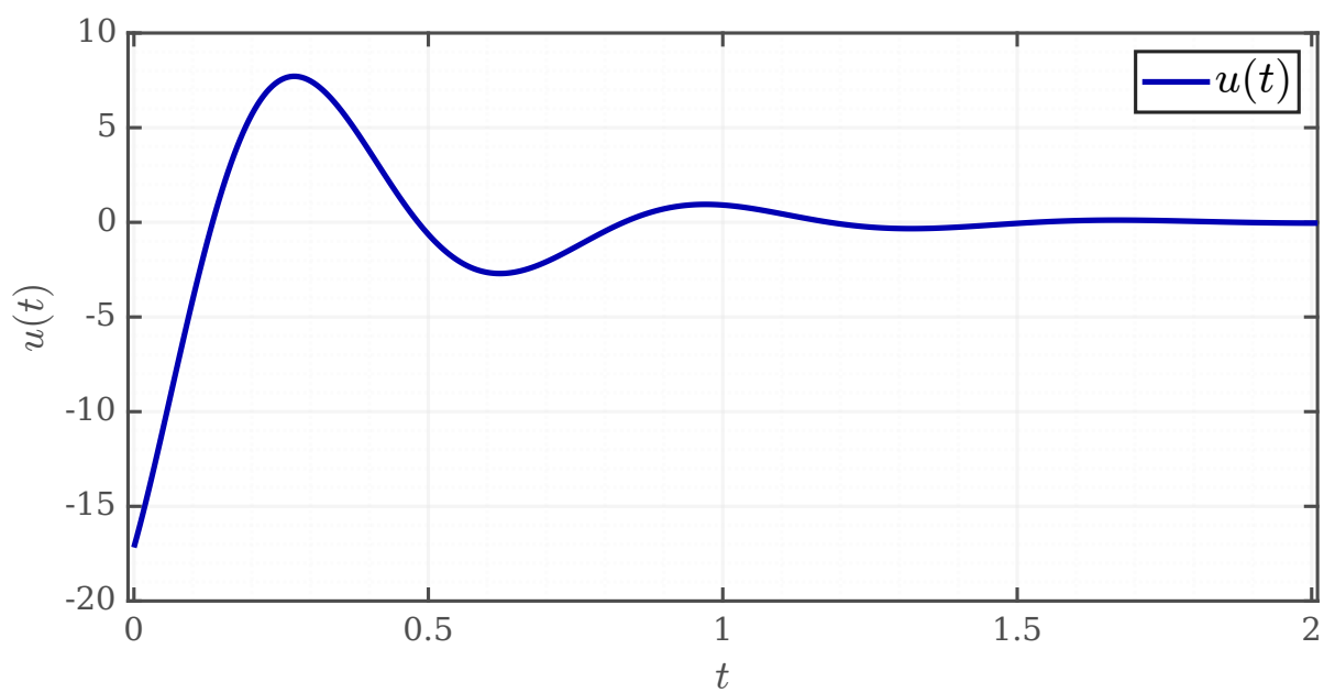
Рисунок 7: Управление u(t)
