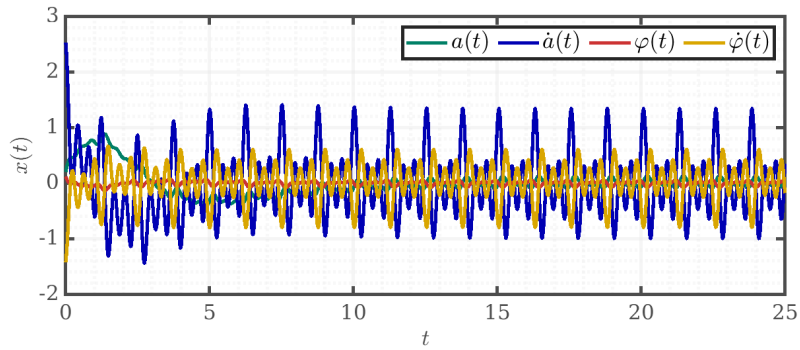
Рис. 117: Линейная модель, неуспешная компенсация
