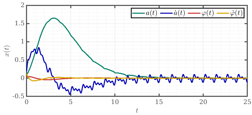
Рис. 118: Нелинейная модель, неуспешная компенсация
