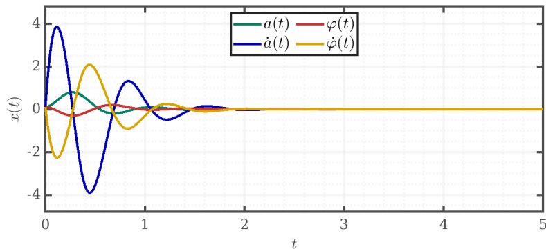
Рис. 90: x(0) = [0.1, 0.1, 0.1, 0.1]^T — успешный
