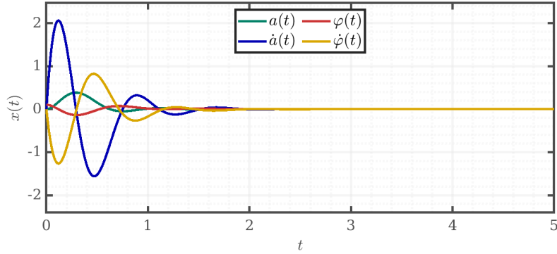
Рис. 88: x(0) = [0, 0, 0.1, 0]^T — успешный
