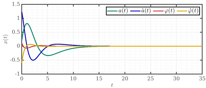
Рис. 115: Линейная модель, успешная компенсация
