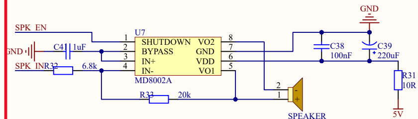
功放电路
