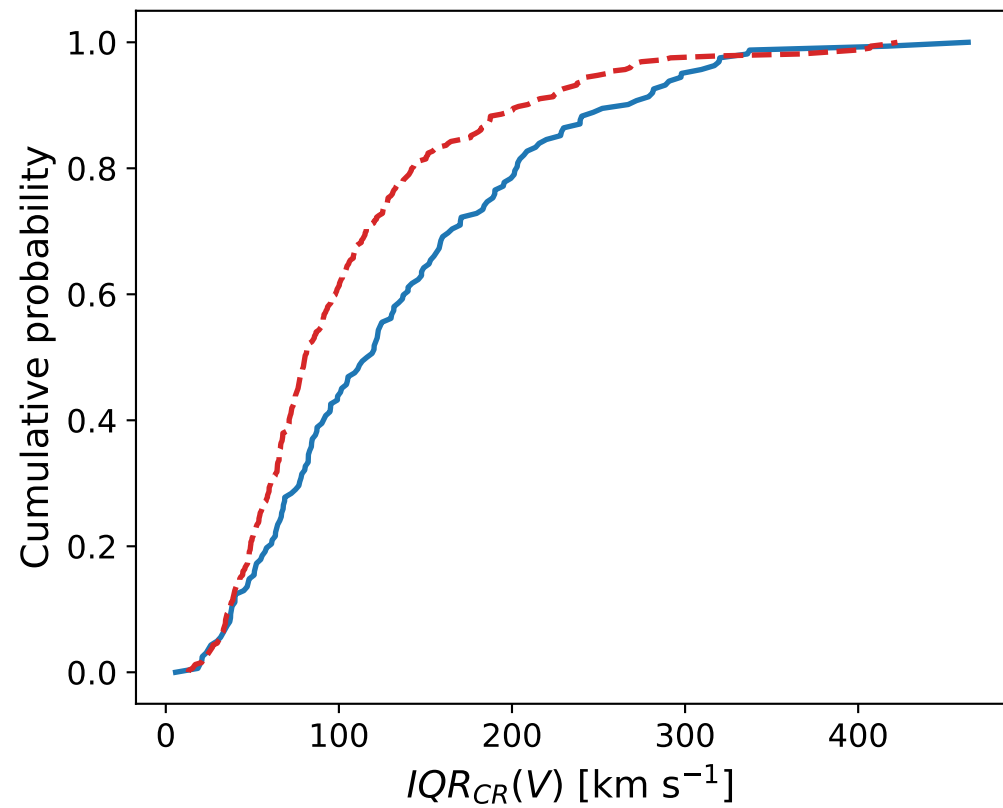
Fast CME ( D=0.208 )
