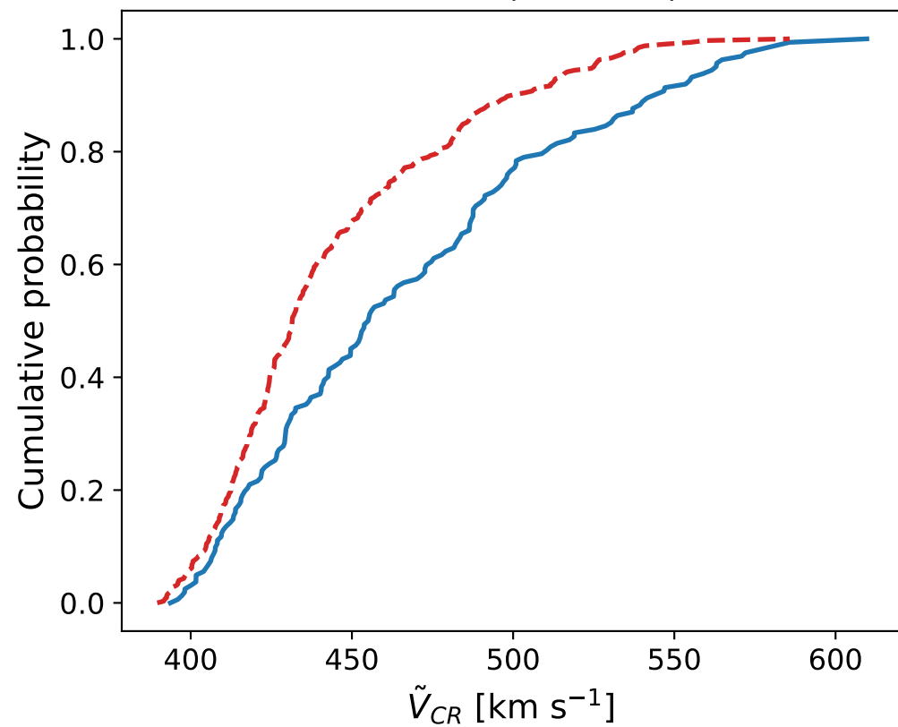
Fast CME ( D=0.238 )
