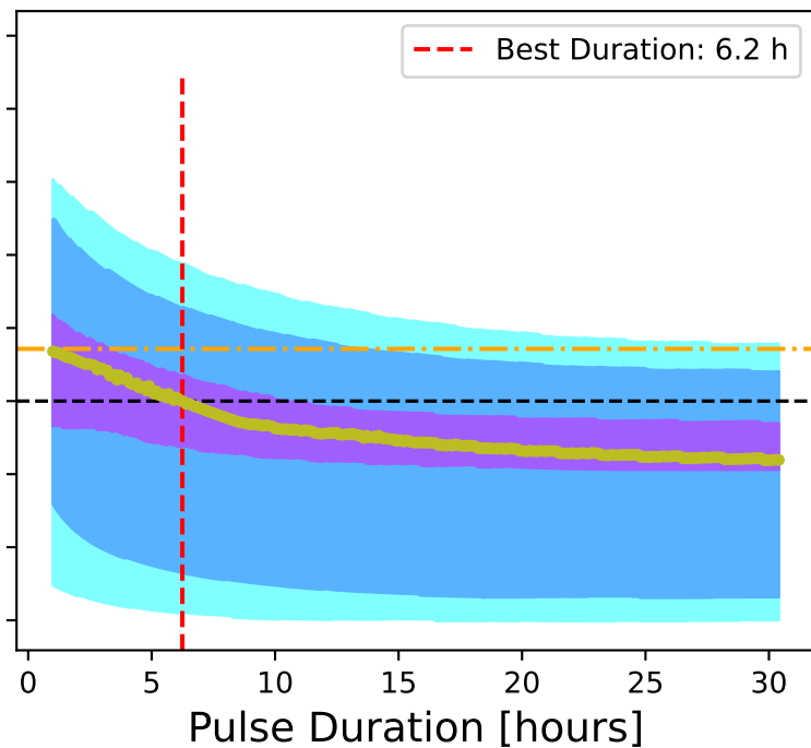
(d) WSA-fcst
