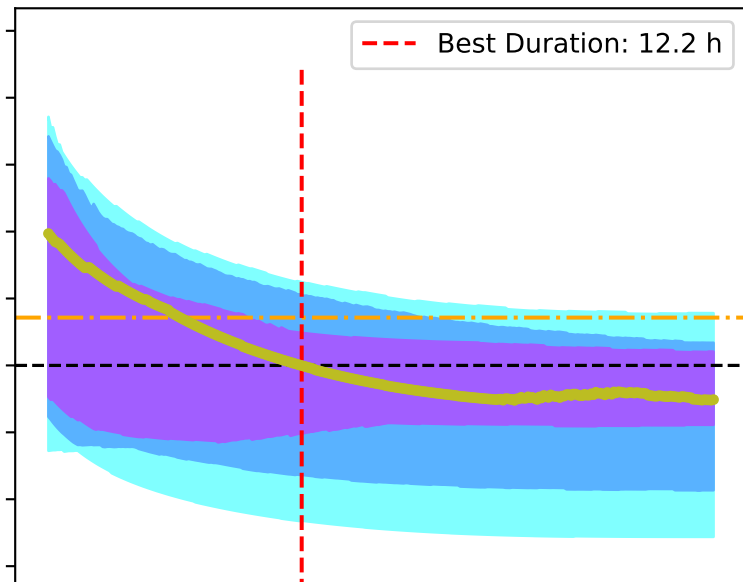
(d) WSA-fcst
