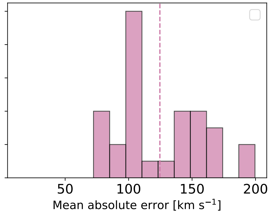
(d) WSA
