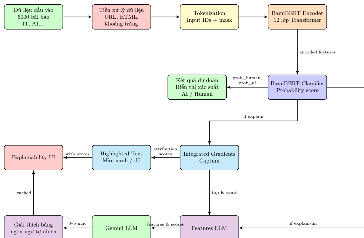
Hình 12: Kiến trúc hệ thống
