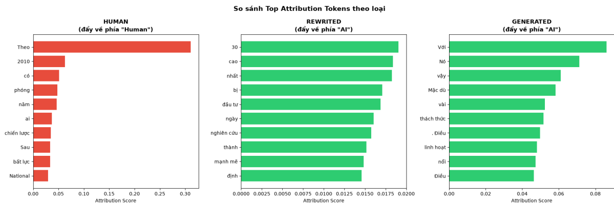
Hình 35: Attribution score của các token tương ứng với ba phương pháp tạo dữ liệu
