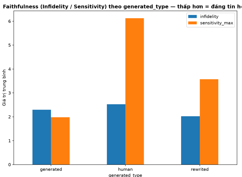
Hình 34: Độ bất trung thực và Độ ổn định
