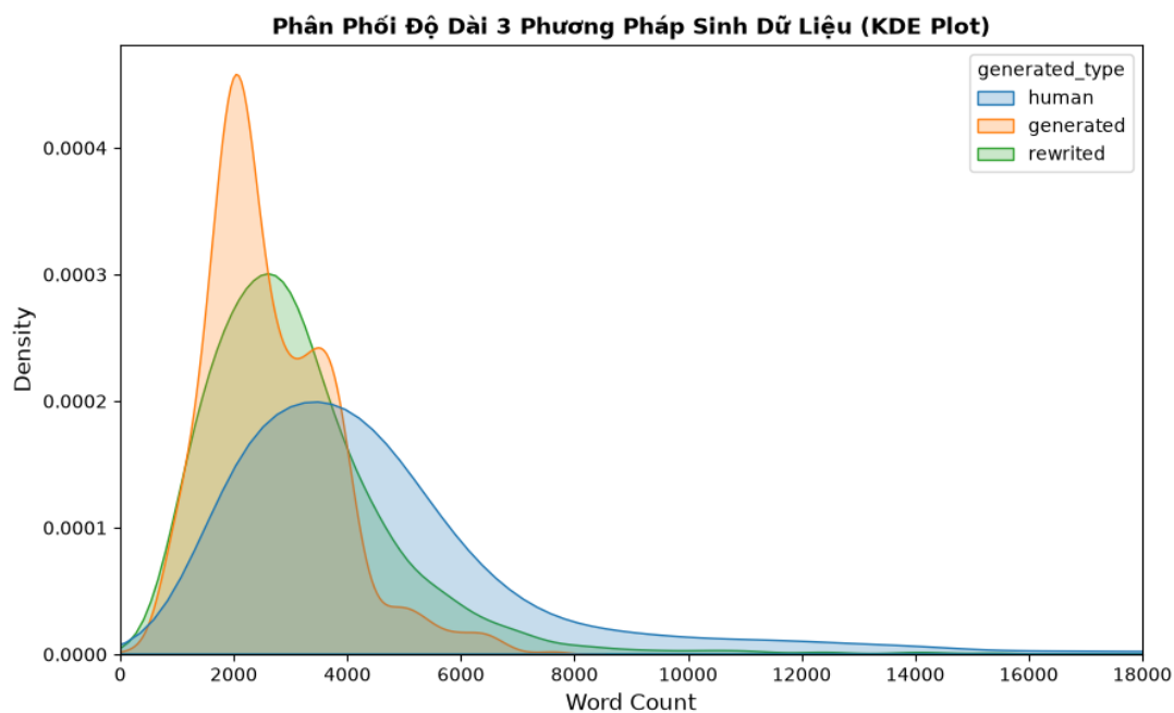
Hình 16: Phân bố độ dài của các phương pháp tạo sinh dữ liệu
