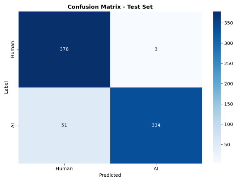
Hình 31: Ma trận sai lầm
