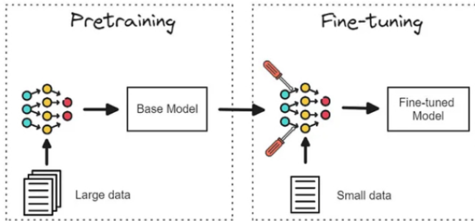
Hình 7: Quá trình fine-tuning
