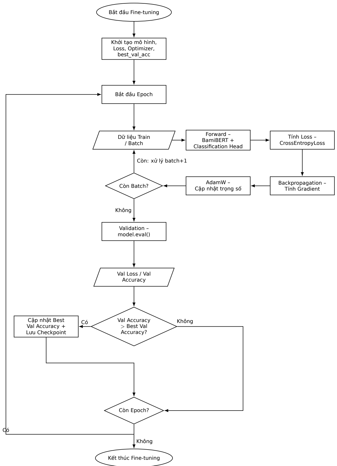
Hình 21: Quá trình fine-tuning
