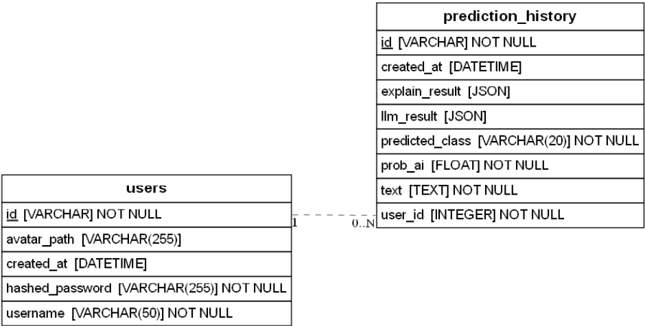
Hình 23: Lược đồ trực quan hóa CSDL
