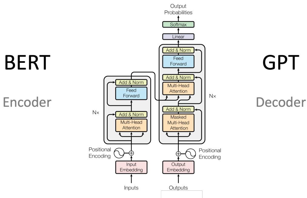
Hình 3: Kiến trúc mô hình Transformer
