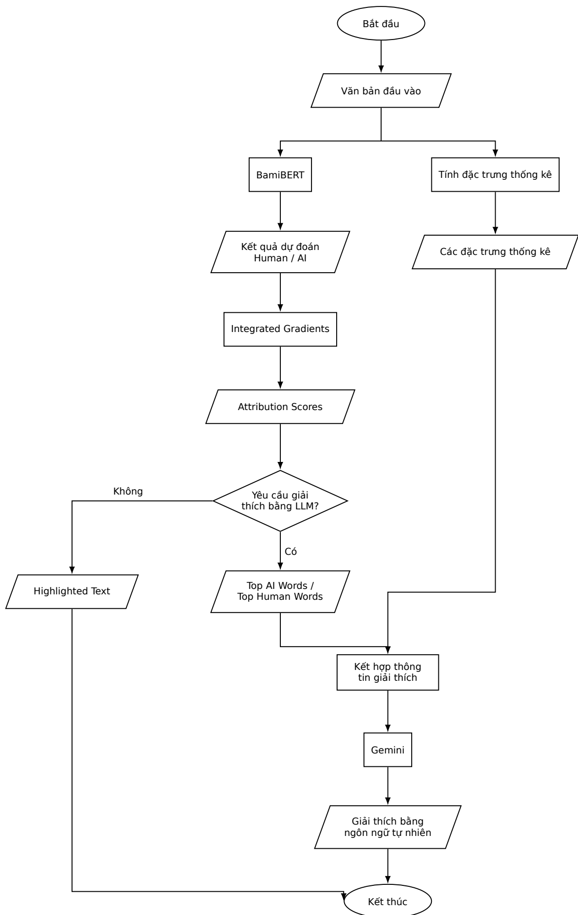
Hình 22: Quá trình đưa ra giải thích
