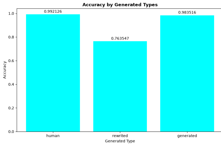
Hình 32: Độ chính xác của ba phương pháp sinh dữ liệu
