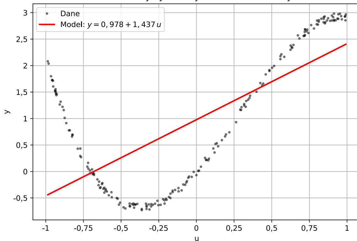
Charakterystyka statyczna - model liniowy
