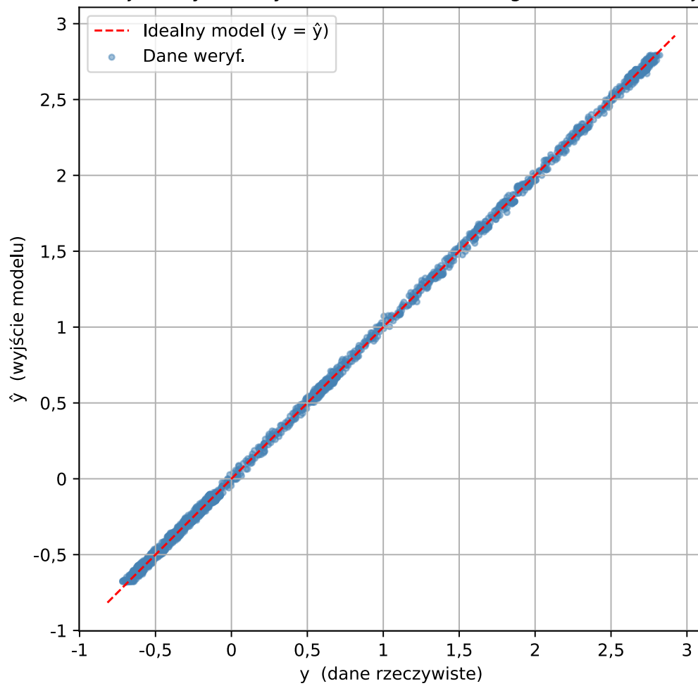
Relacja danych weryf. vs NARX(nA=16, deg=4) - z rekurencją
