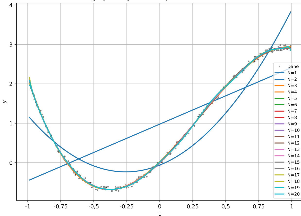
Charakterystyki statyczne - wszystkie modele wielomianowe
