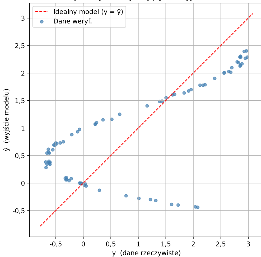
Relacja danych weryfikujących i wyjścia modelu
