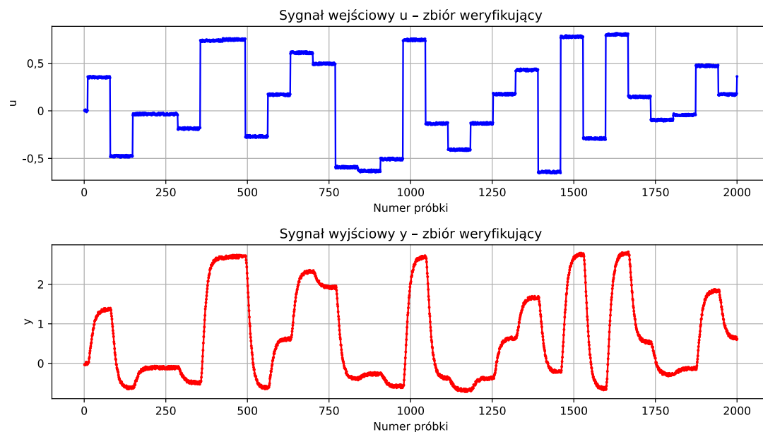
Dane dynamiczne - zbiór weryfikujący (N = 2000)
