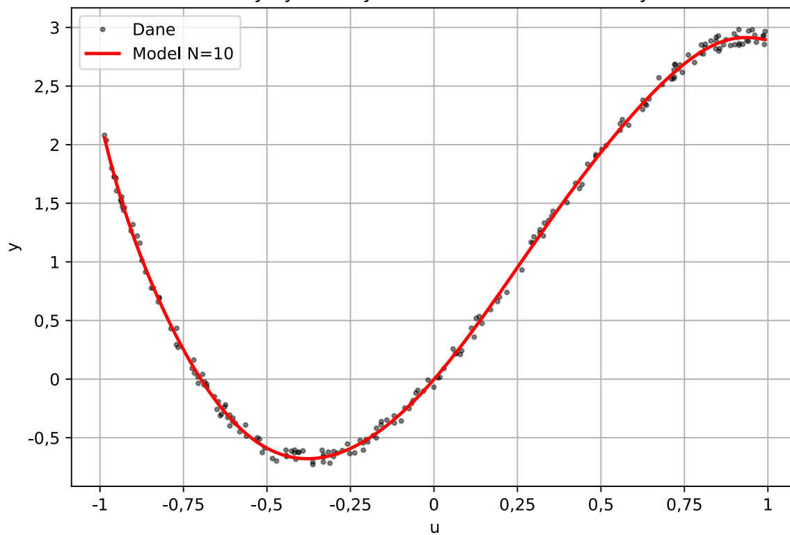
Charakterystyka statyczna - model wielomianowy N=10
