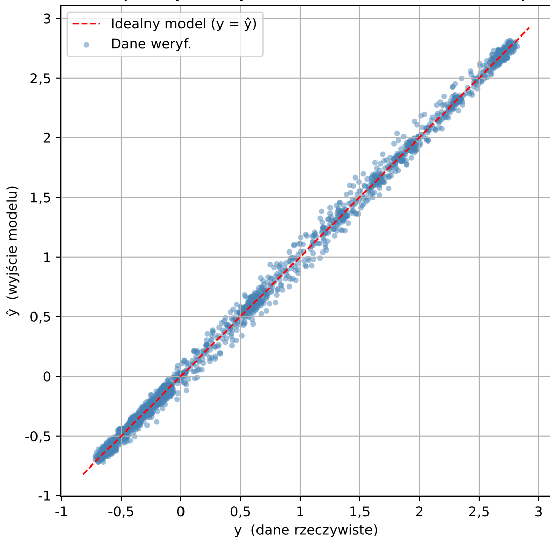
Relacja danych weryf. vs model ARX(1) - bez rekurencji
