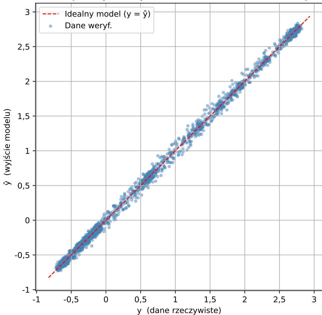
Relacja danych weryf. vs model ARX(2) - bez rekurencji
