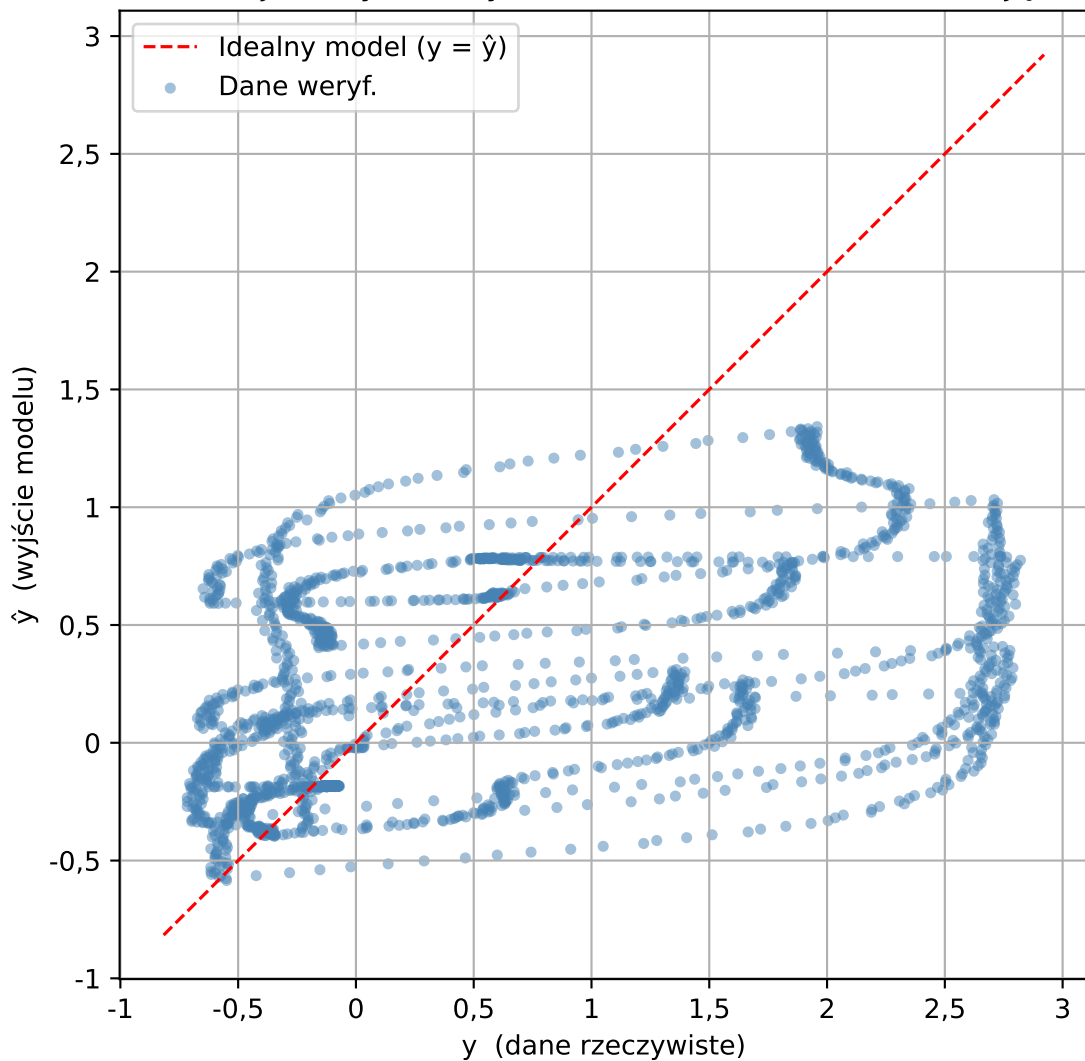
Relacja danych weryf. vs model ARX(2) - z rekurencją
