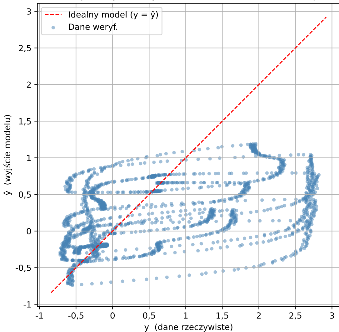
Relacja danych weryf. vs model ARX(3) - z rekurencją
