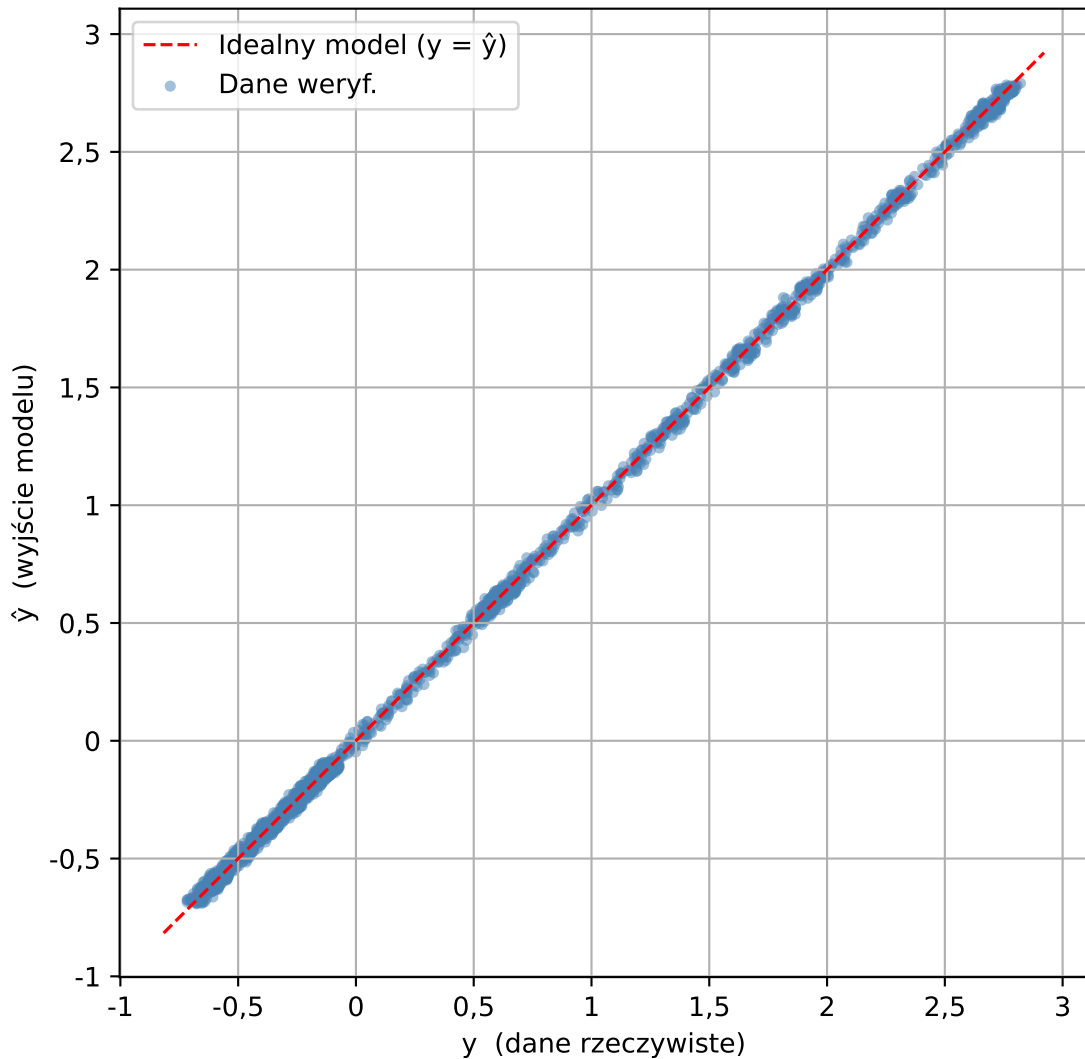
Relacja danych weryf. vs NARX( n_A=13 , \text{deg}=3 ) - bez rekurencji
