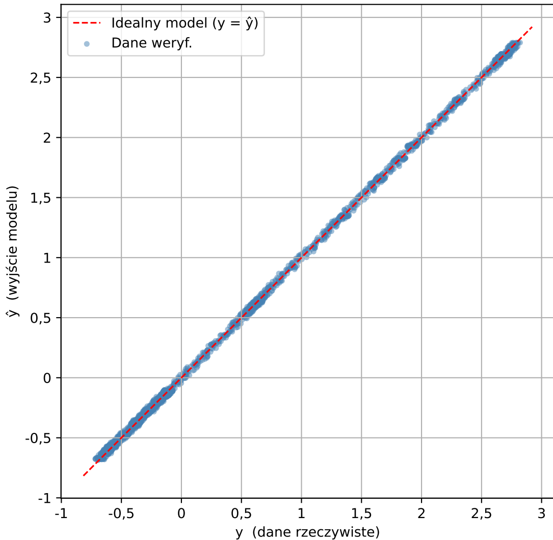
Relacja danych weryf. vs NARX(nA=13, deg=4) - z rekurencją
