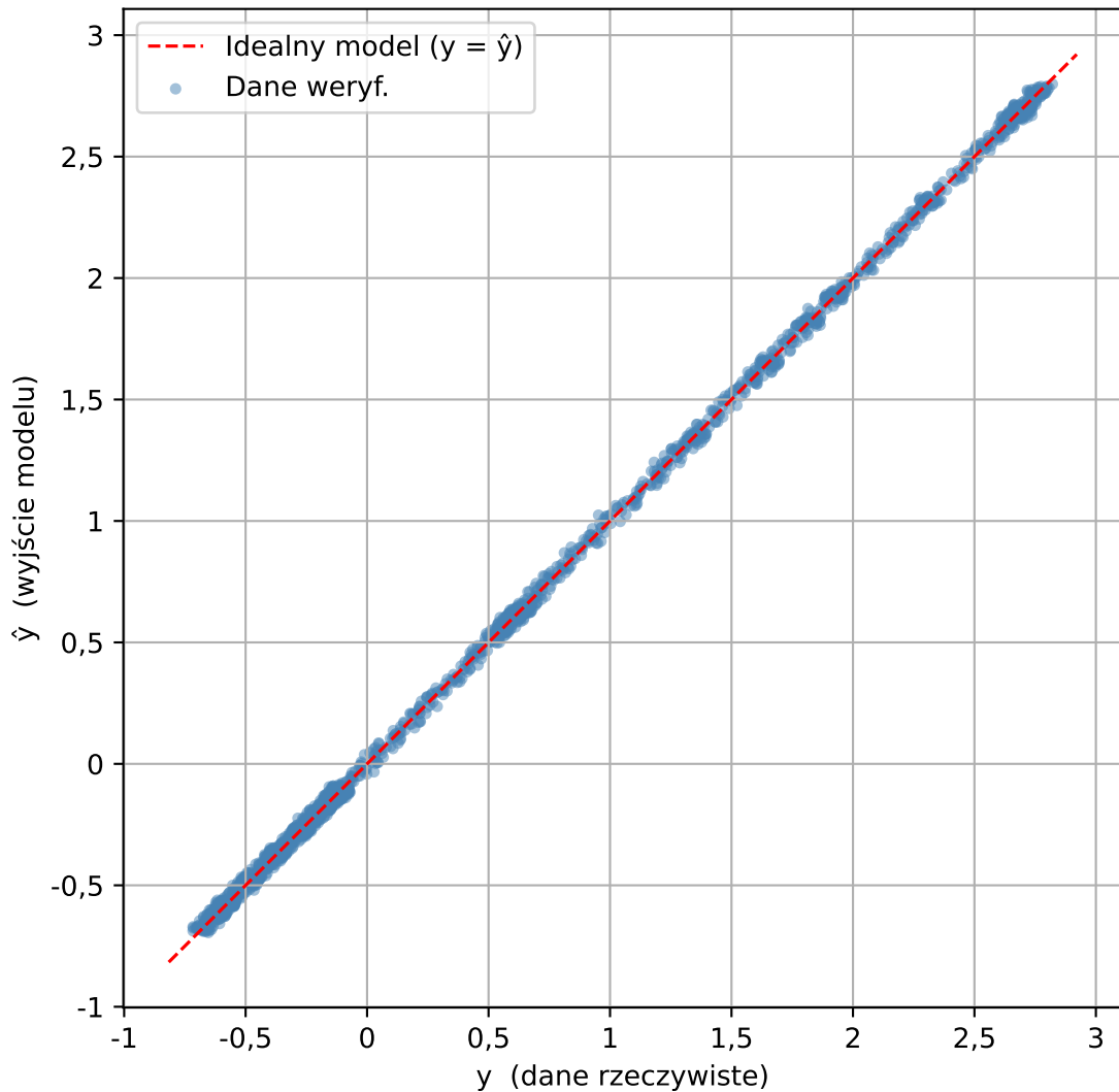
Relacja danych weryf. vs NARX( n_A=13 , \text{deg}=5 ) - bez rekurencji
