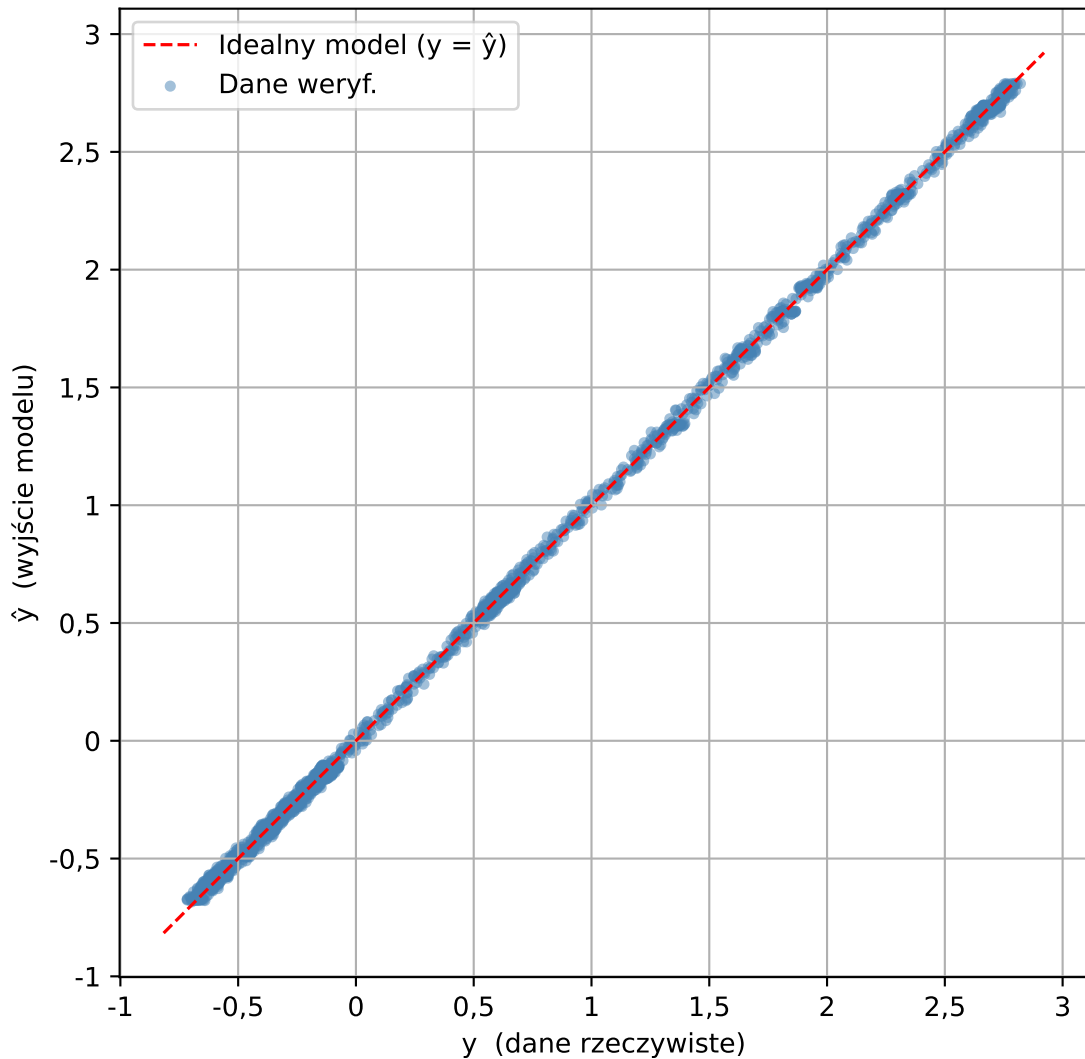
Relacja danych weryf. vs NARX(nA=13, deg=5) - z rekurencją
