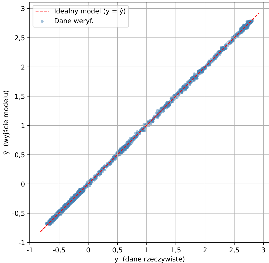
Relacja danych weryf. vs NARX( n_A=13 , \text{deg}=6 ) - bez rekurencji
