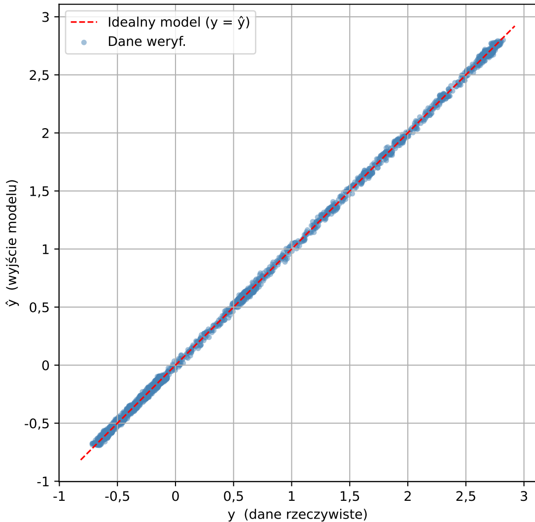
Relacja danych weryf. vs NARX( n_A=14 , \text{deg}=4 ) - bez rekurencji
