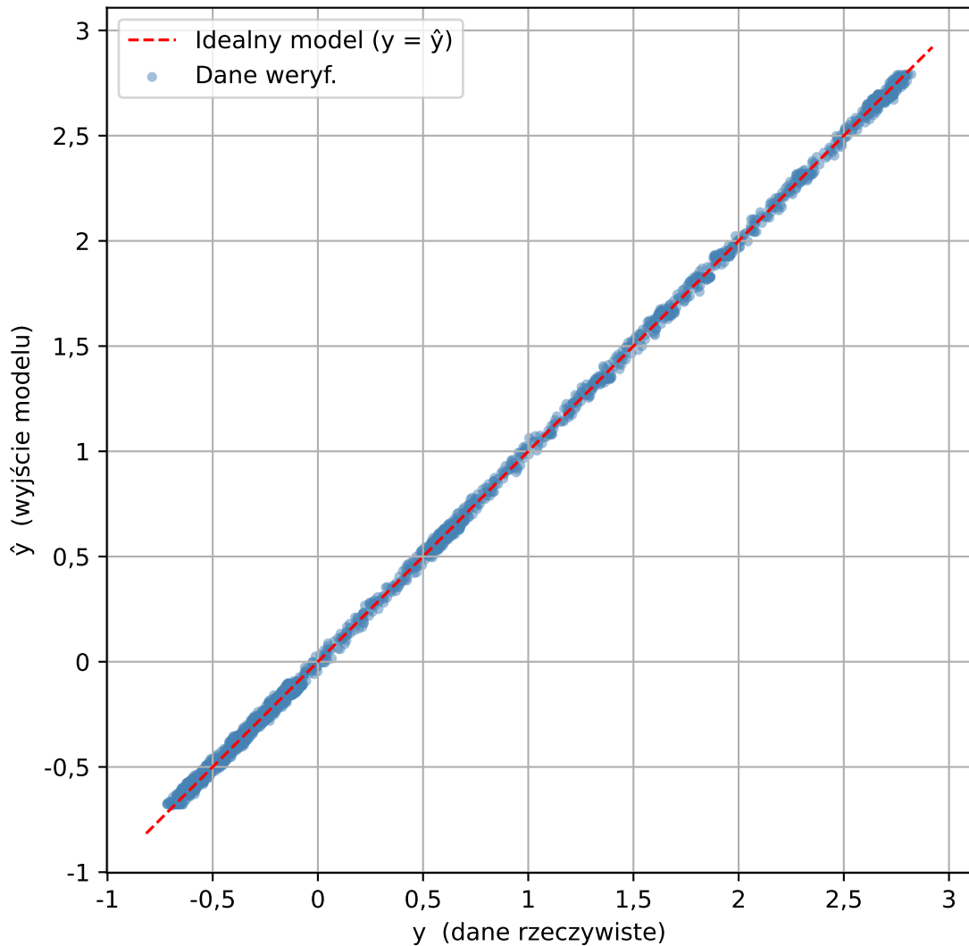
Relacja danych weryf. vs NARX(nA=14, deg=4) - z rekurencją
