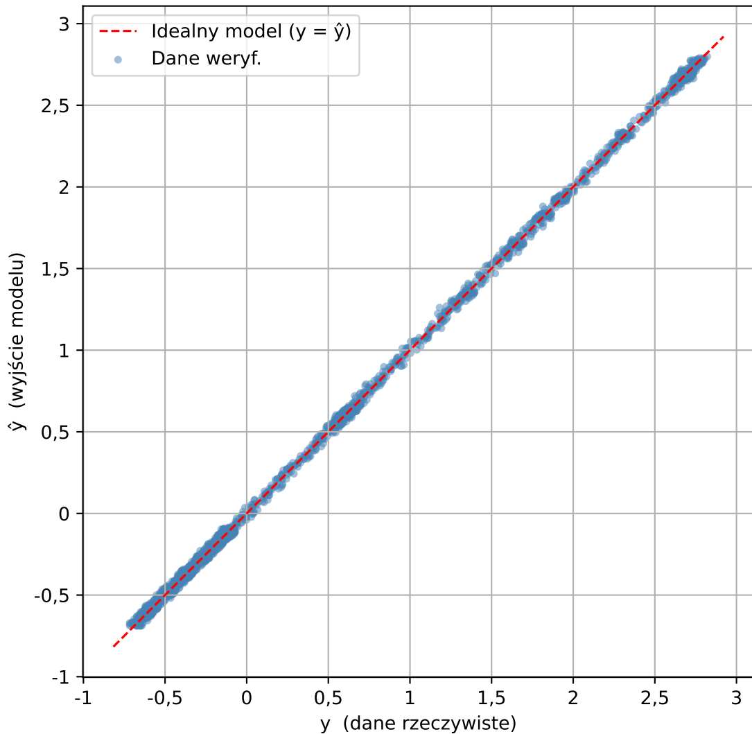
Relacja danych weryf. vs NARX( n_A=14 , \text{deg}=6 ) - bez rekurencji
