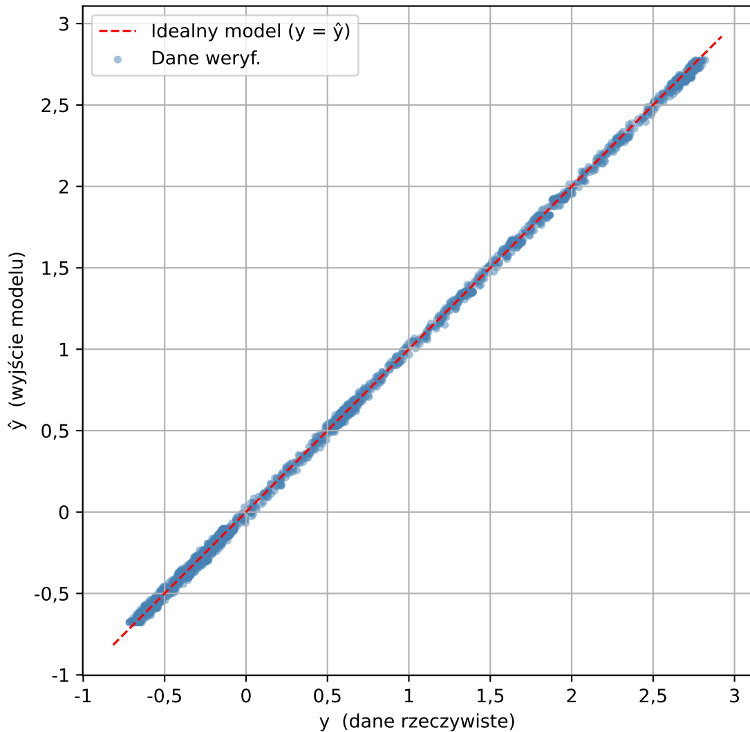
Relacja danych weryf. vs NARX(nA=15, deg=3) - z rekurencją
