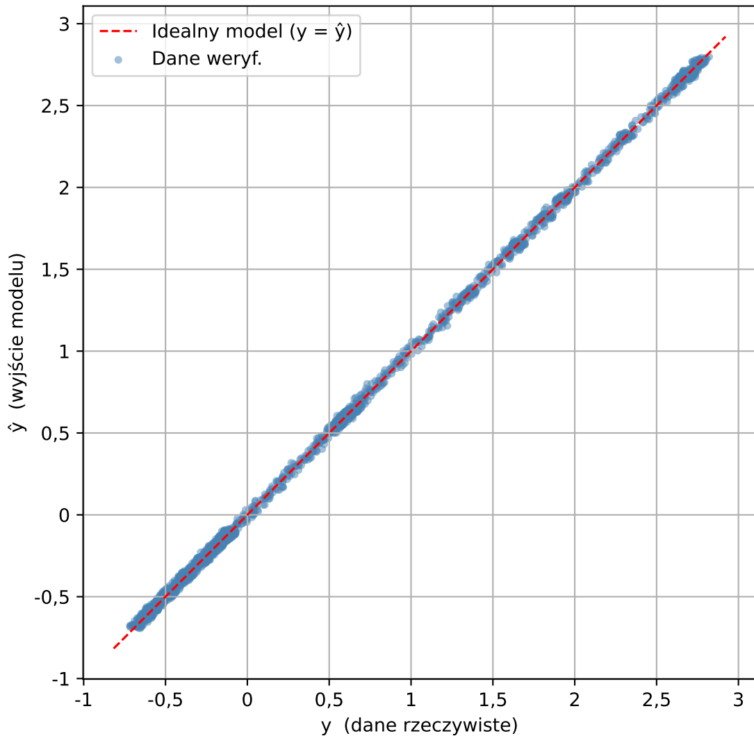
Relacja danych weryf. vs NARX( n_A=15 , \text{deg}=4 ) - bez rekurencji
