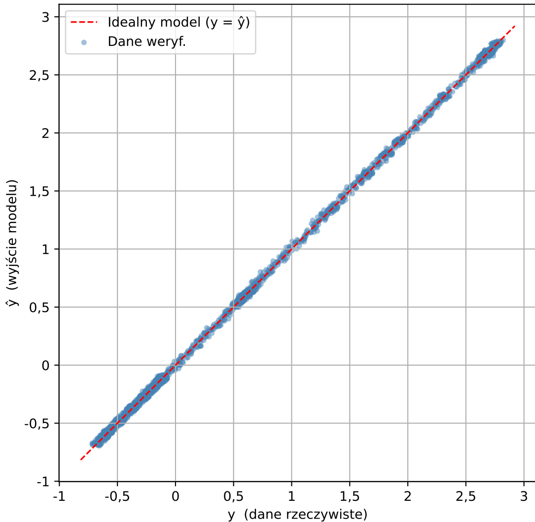
Relacja danych weryf. vs NARX( n_A=15 , \text{deg}=5 ) - bez rekurencji
