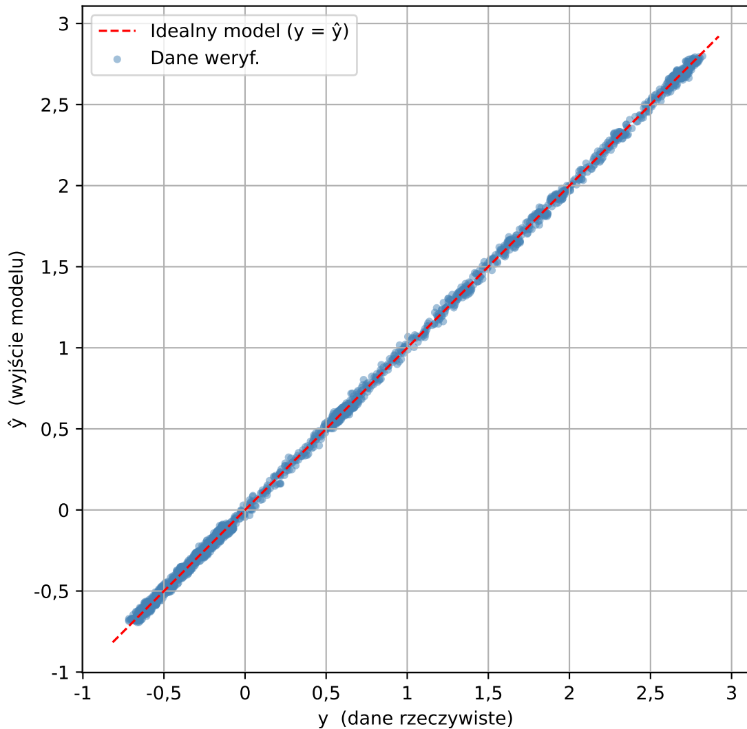
Relacja danych weryf. vs NARX( n_A=16 , \text{deg}=5 ) - bez rekurencji
