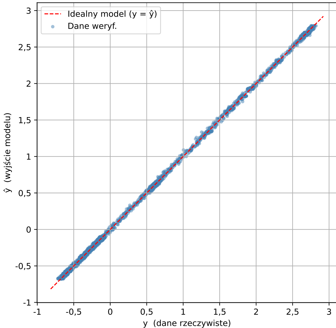
Relacja danych weryf. vs NARX(nA=16, deg=6) - z rekurencją
