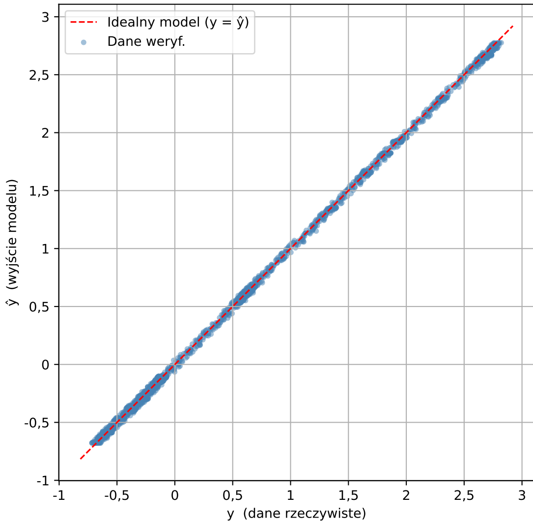
Relacja danych weryf. vs NARX(nA=17, deg=3) - z rekurencją
