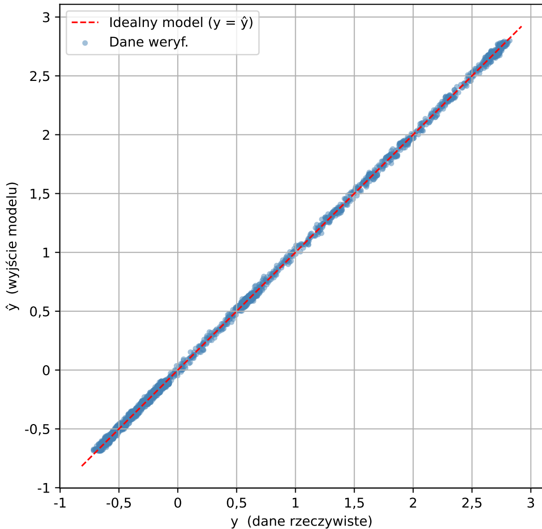
Relacja danych weryf. vs NARX( n_A=17 , \text{deg}=4 ) - bez rekurencji
