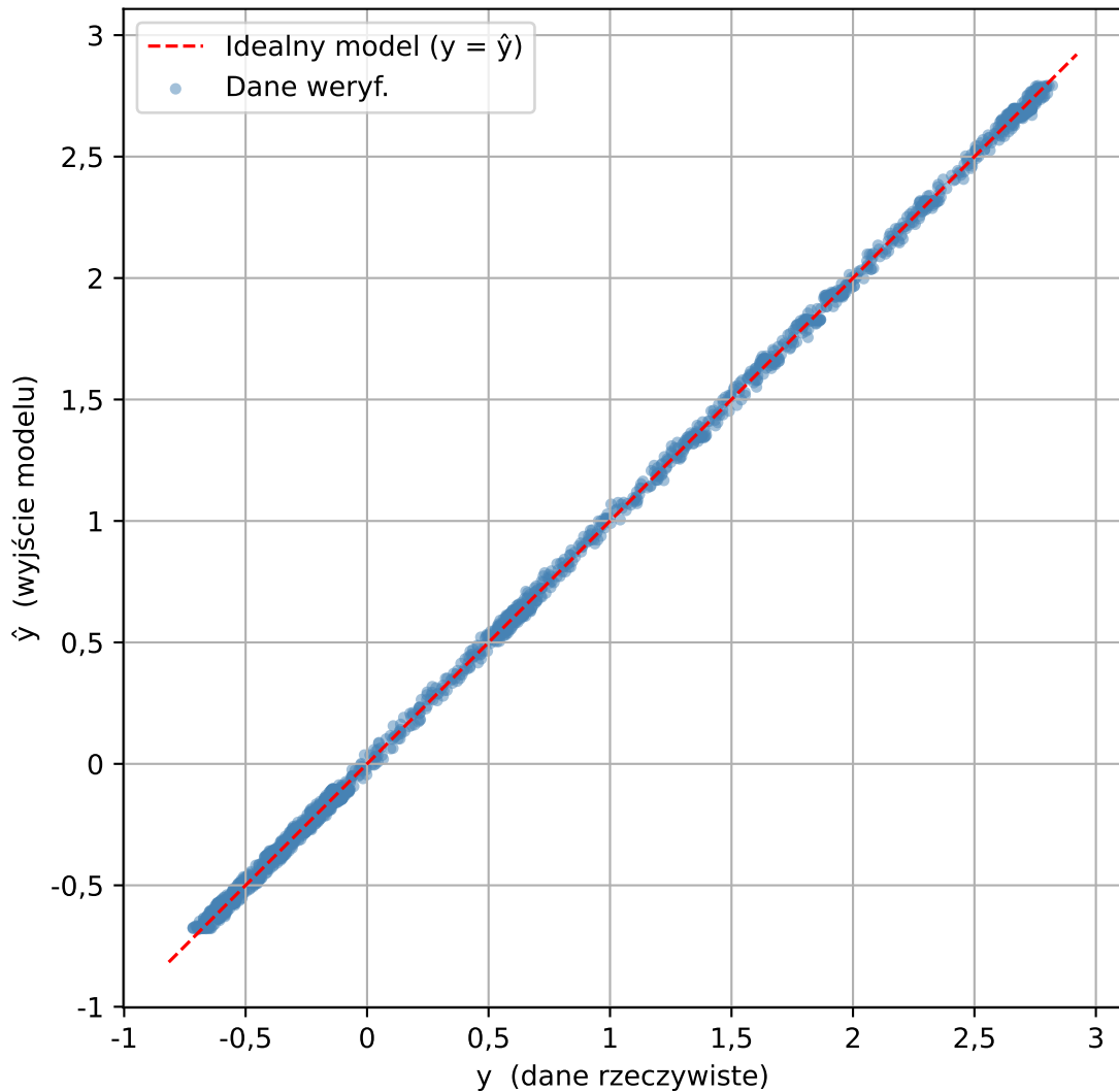
Relacja danych weryf. vs NARX(nA=17, deg=4) - z rekurencją
