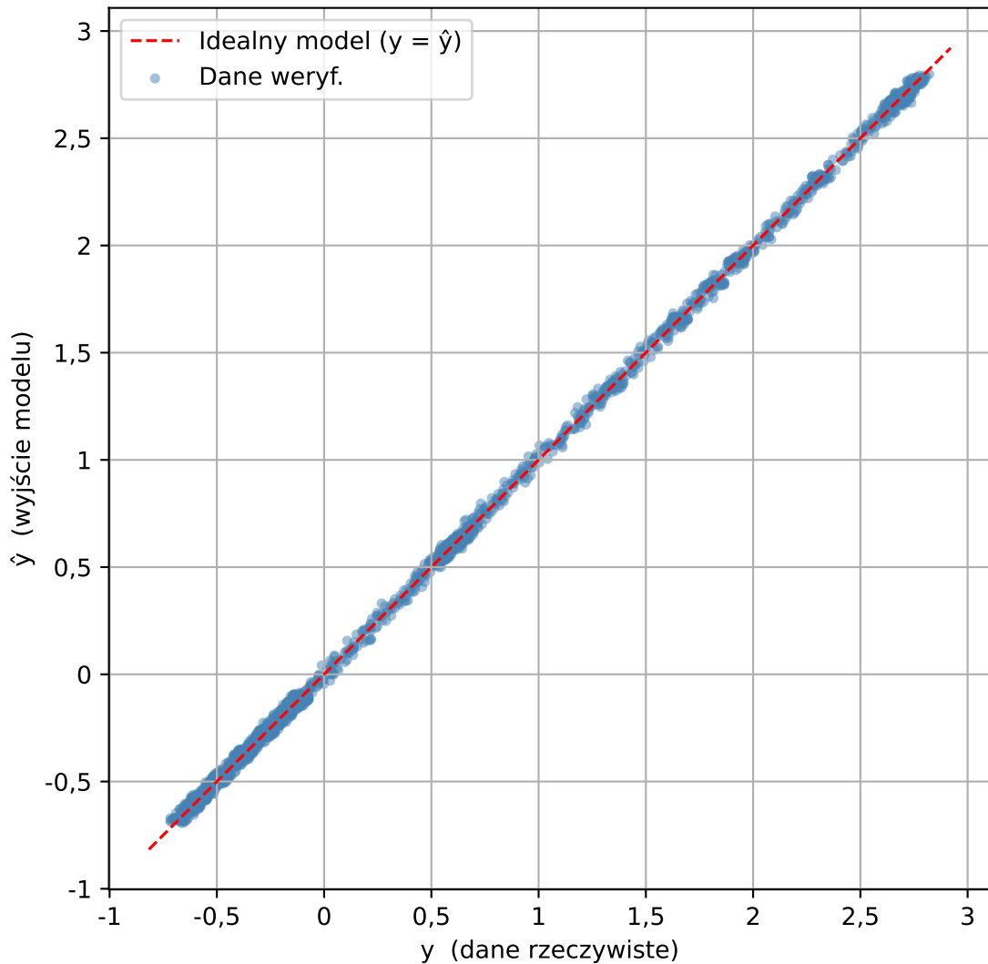
Relacja danych weryf. vs NARX( n_A=17 , \text{deg}=5 ) - bez rekurencji
