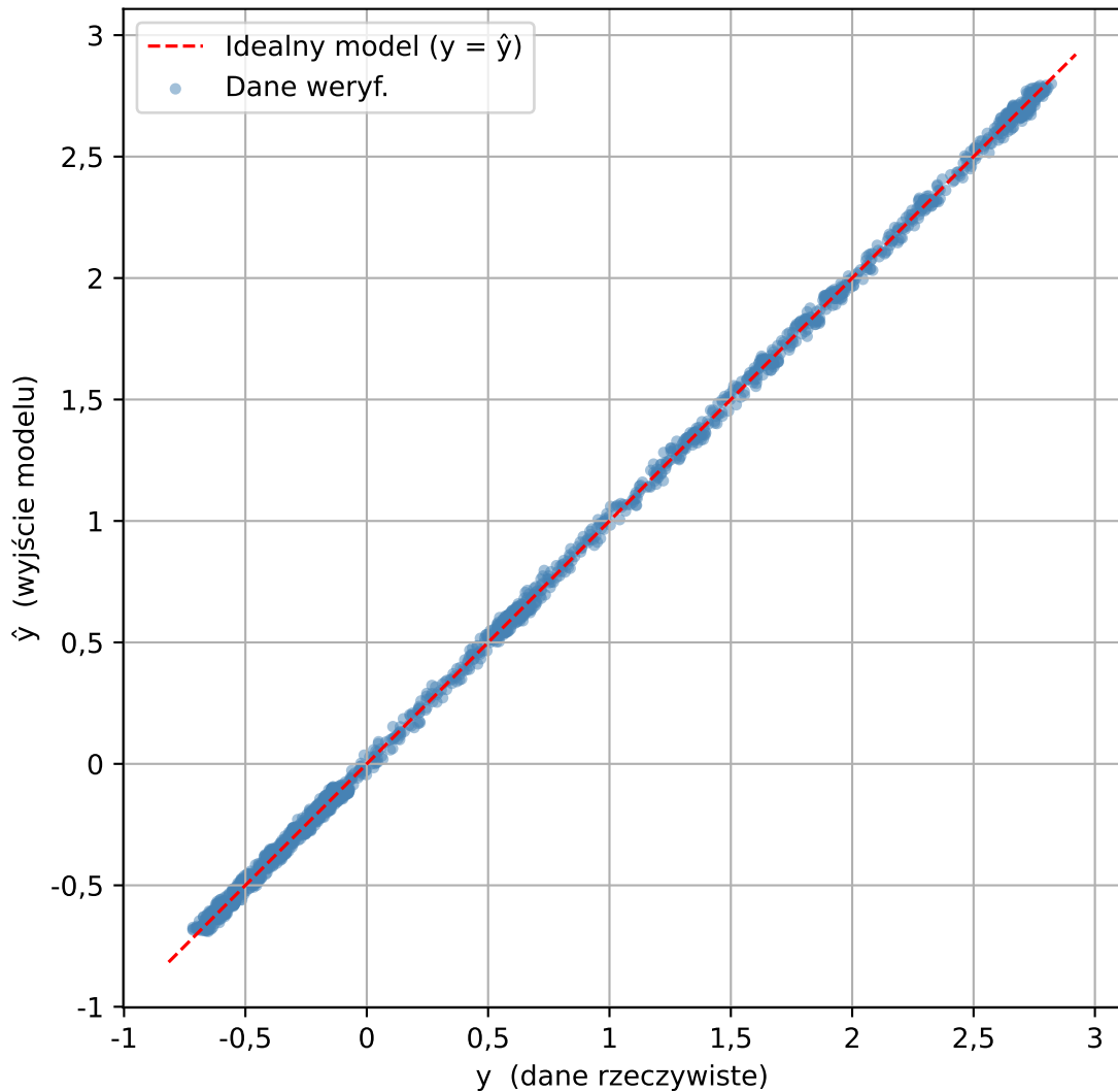
Relacja danych weryf. vs NARX( n_A=18 , \text{deg}=4 ) - bez rekurencji
