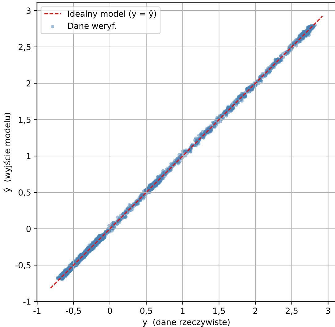
Relacja danych weryf. vs NARX( n_A=18 , \text{deg}=5 ) - bez rekurencji
