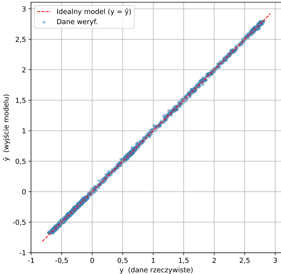
Relacja danych weryf. vs NARX(nA=18, deg=6) - z rekurencją
