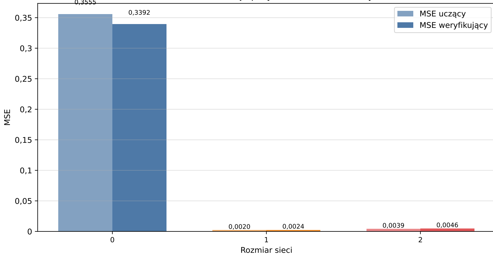
Porównanie MSE najlepszych modeli neuronowych
