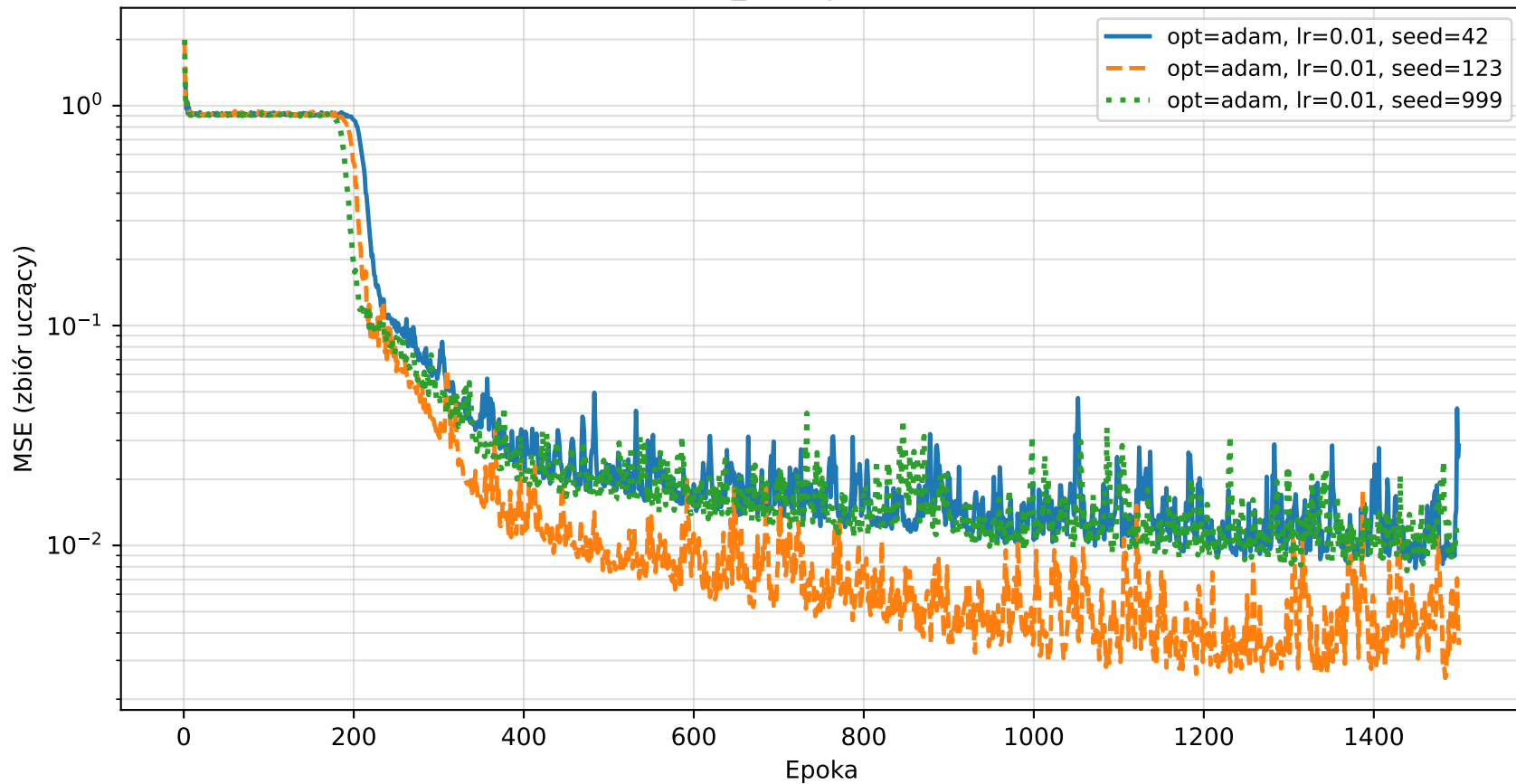
Krzywe uczenia - zbyt_duza | zmiana punktu startowego
