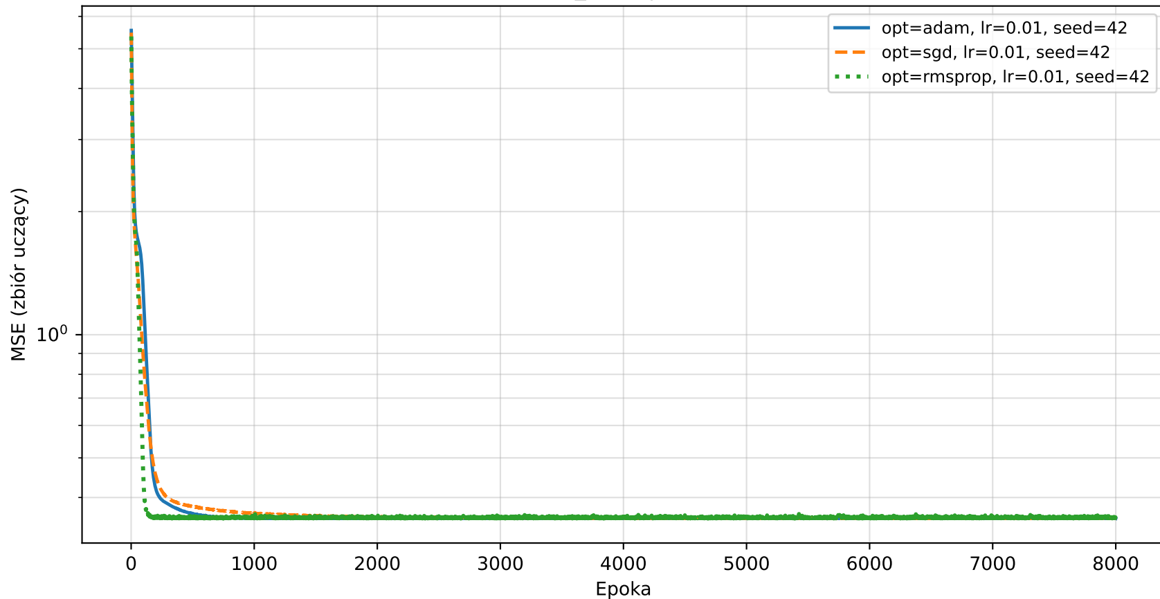
Krzywe uczenia - zbyt_mala | zmiana optymalizatora
