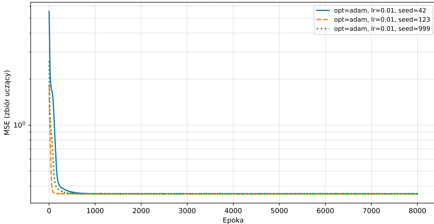
Krzywe uczenia - zbyt_mala | zmiana punktu startowego
