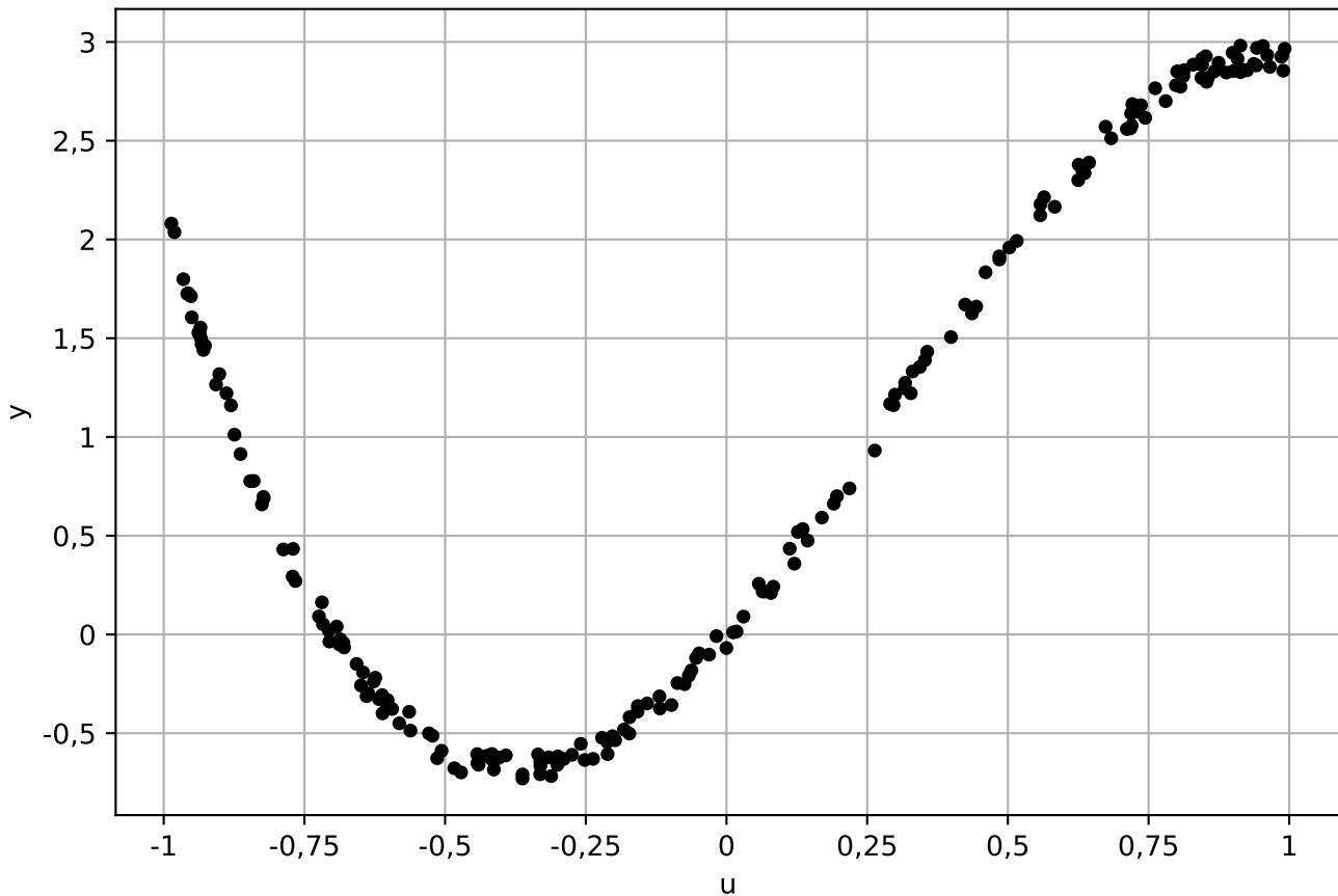
Charakterystyka statyczna y = f(u) - wszystkie dane
