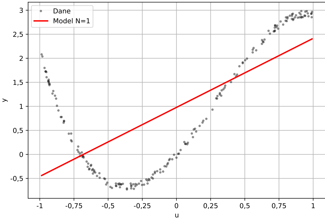
Charakterystyka statyczna - model wielomianowy N=1
