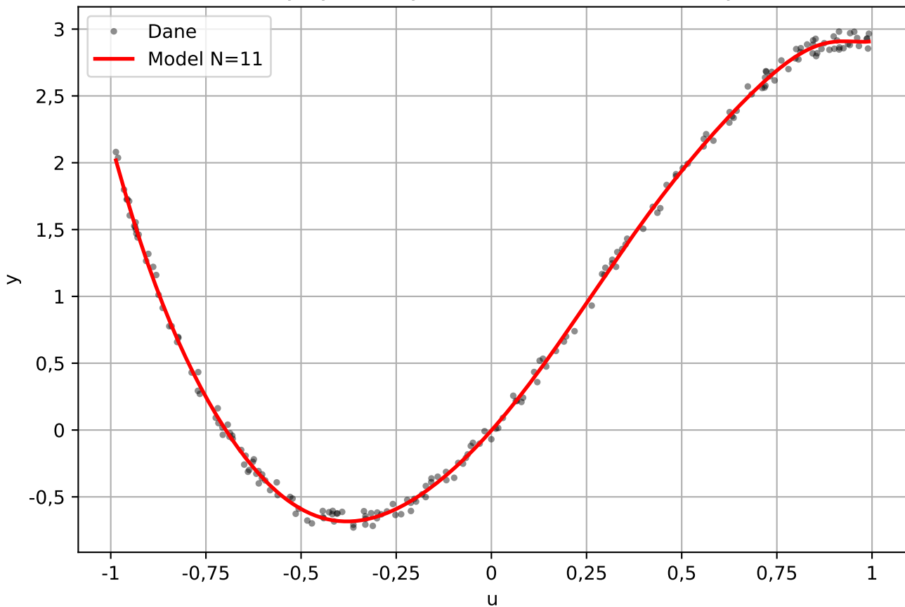
Charakterystyka statyczna - model wielomianowy N=11
