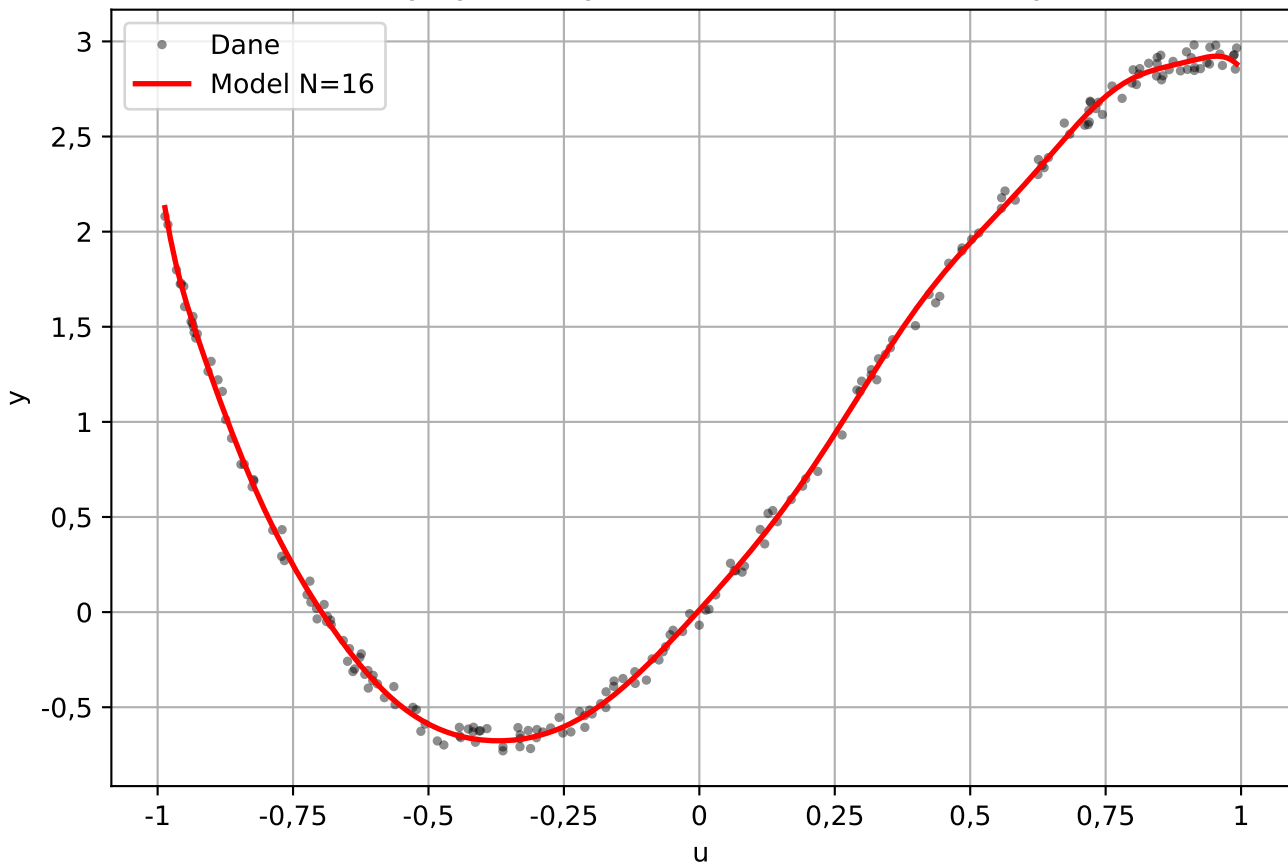
Charakterystyka statyczna - model wielomianowy N=16
