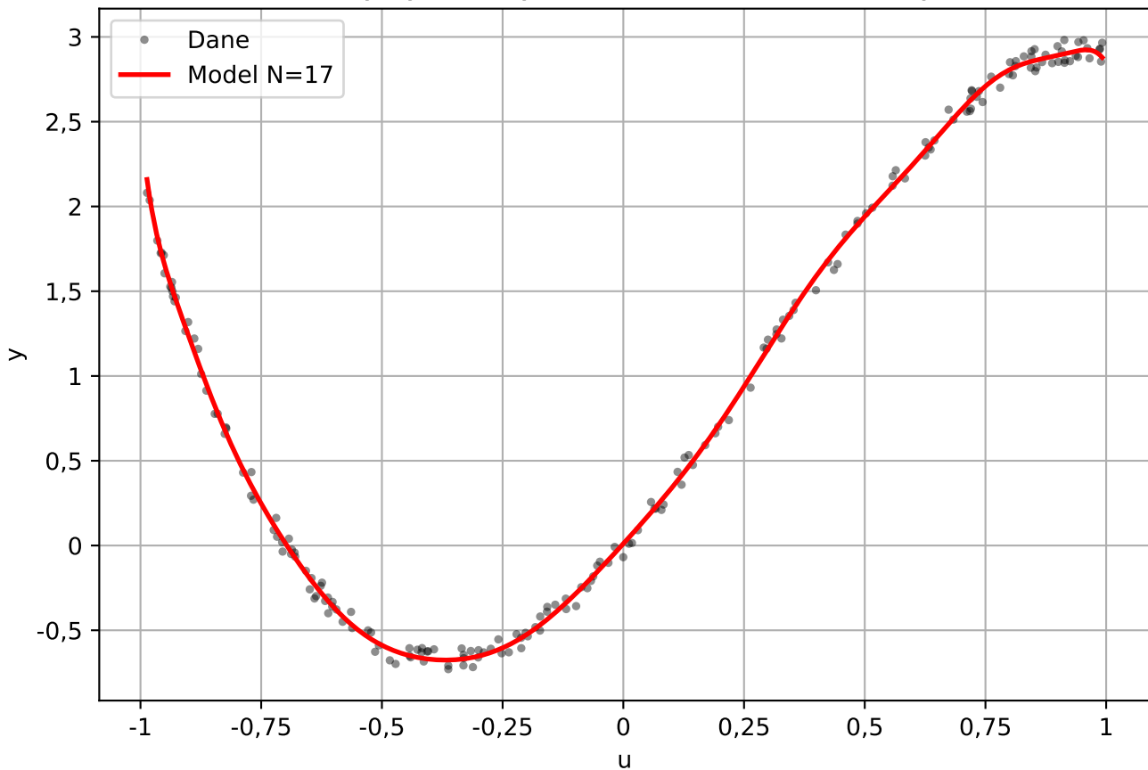
Charakterystyka statyczna - model wielomianowy N=17
