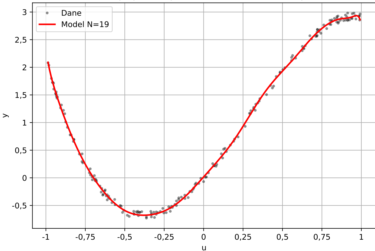
Charakterystyka statyczna - model wielomianowy N=19
