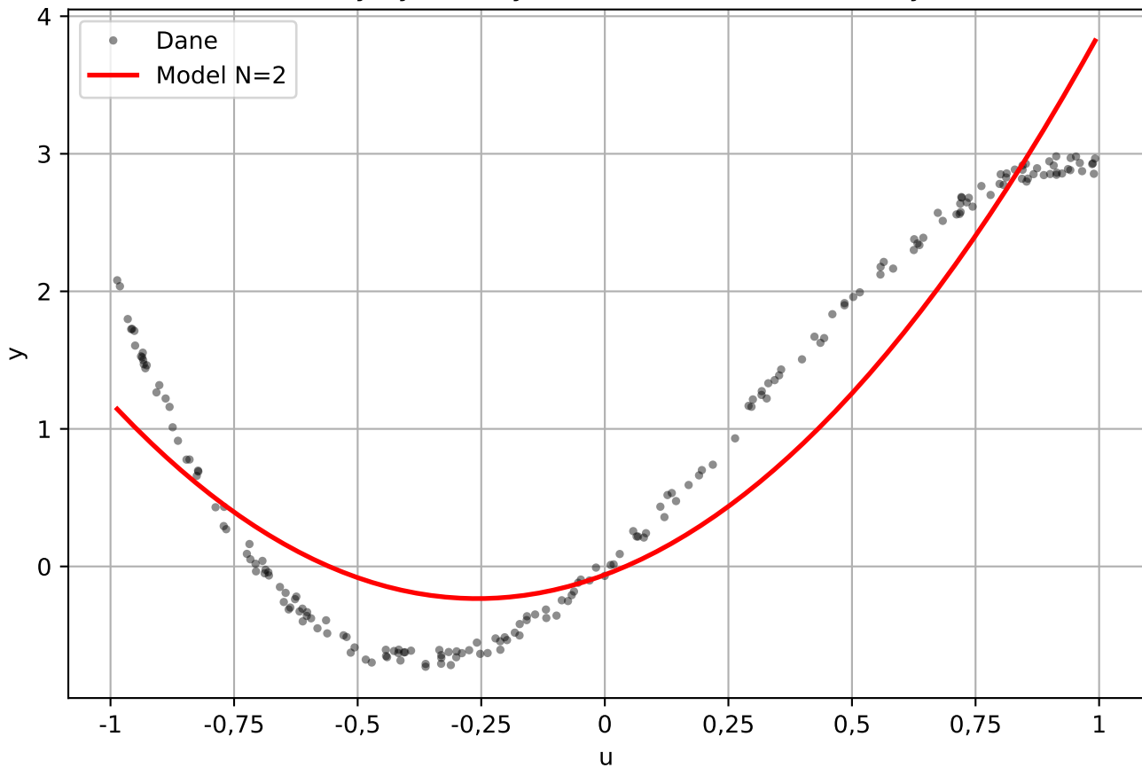
Charakterystyka statyczna - model wielomianowy N=2
