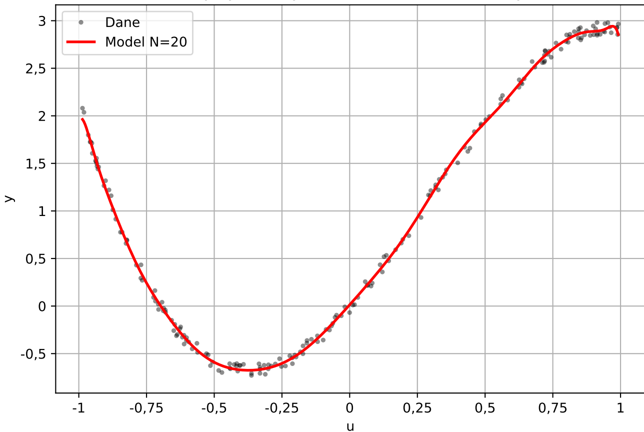
Charakterystyka statyczna - model wielomianowy N=20
