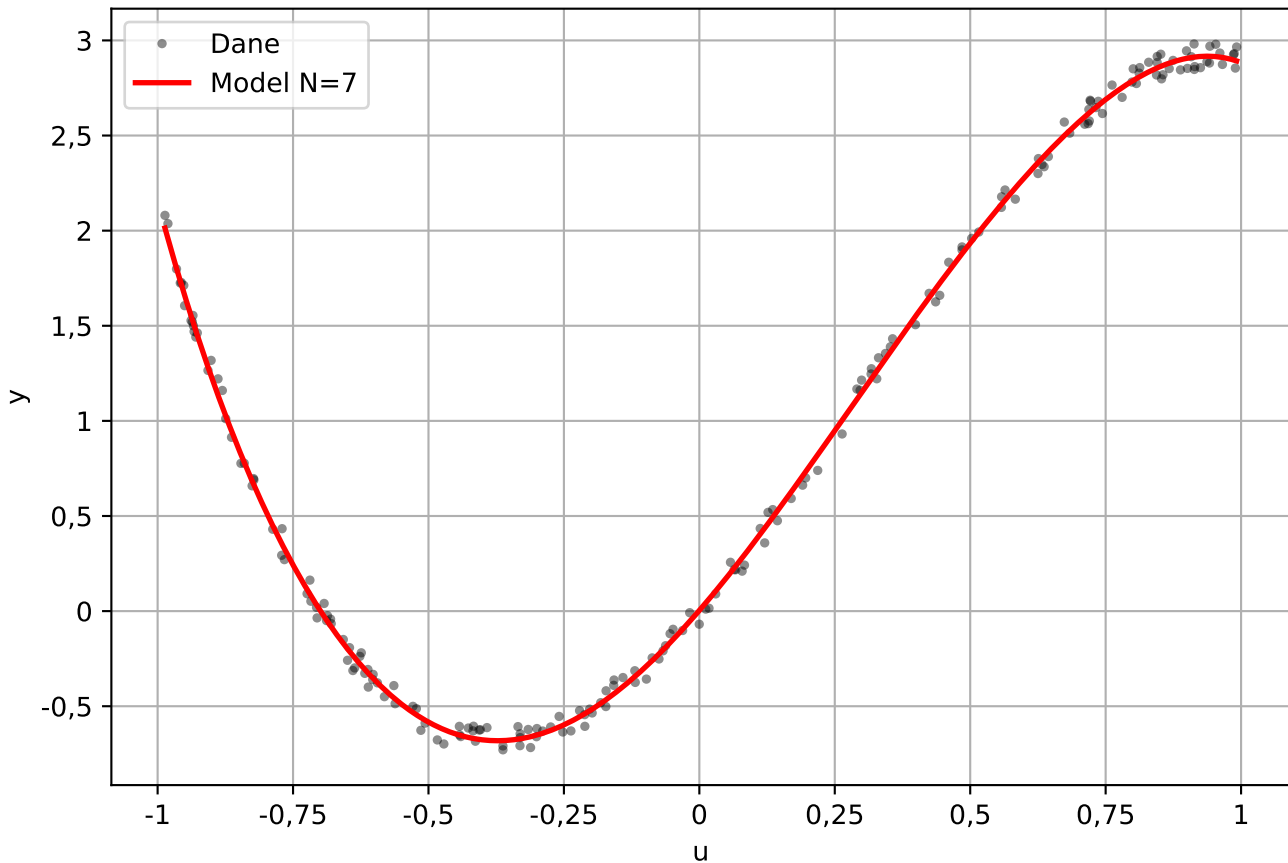
Charakterystyka statyczna - model wielomianowy N=7
