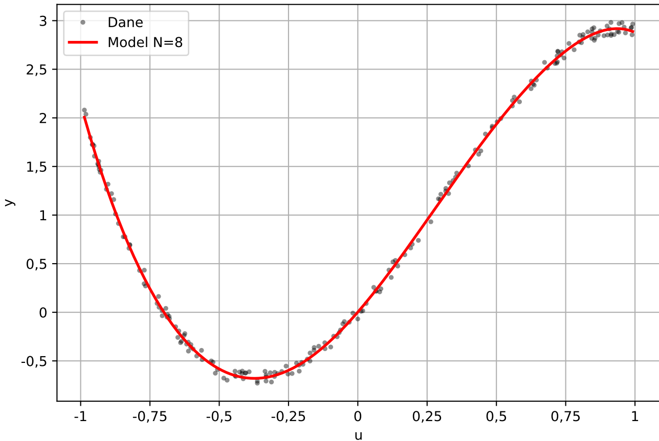
Charakterystyka statyczna - model wielomianowy N=8
