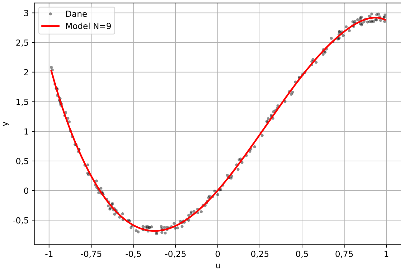
Charakterystyka statyczna - model wielomianowy N=9
