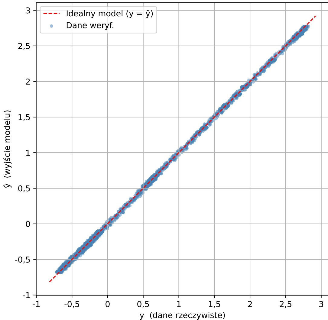
Relacja danych weryf. vs NARX(nA=13, deg=3) - z rekurencją
