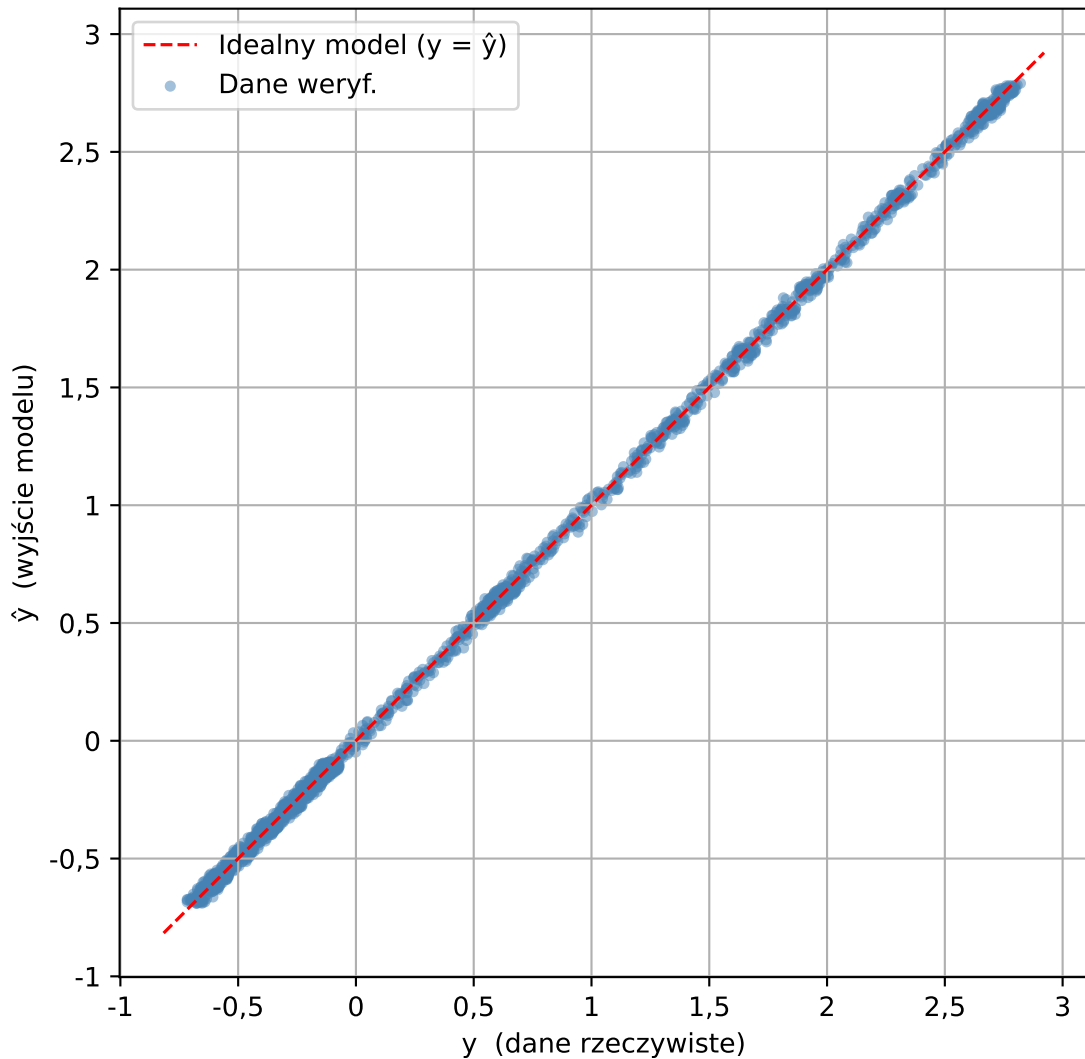
Relacja danych weryf. vs NARX( n_A=14 , \text{deg}=3 ) - bez rekurencji
