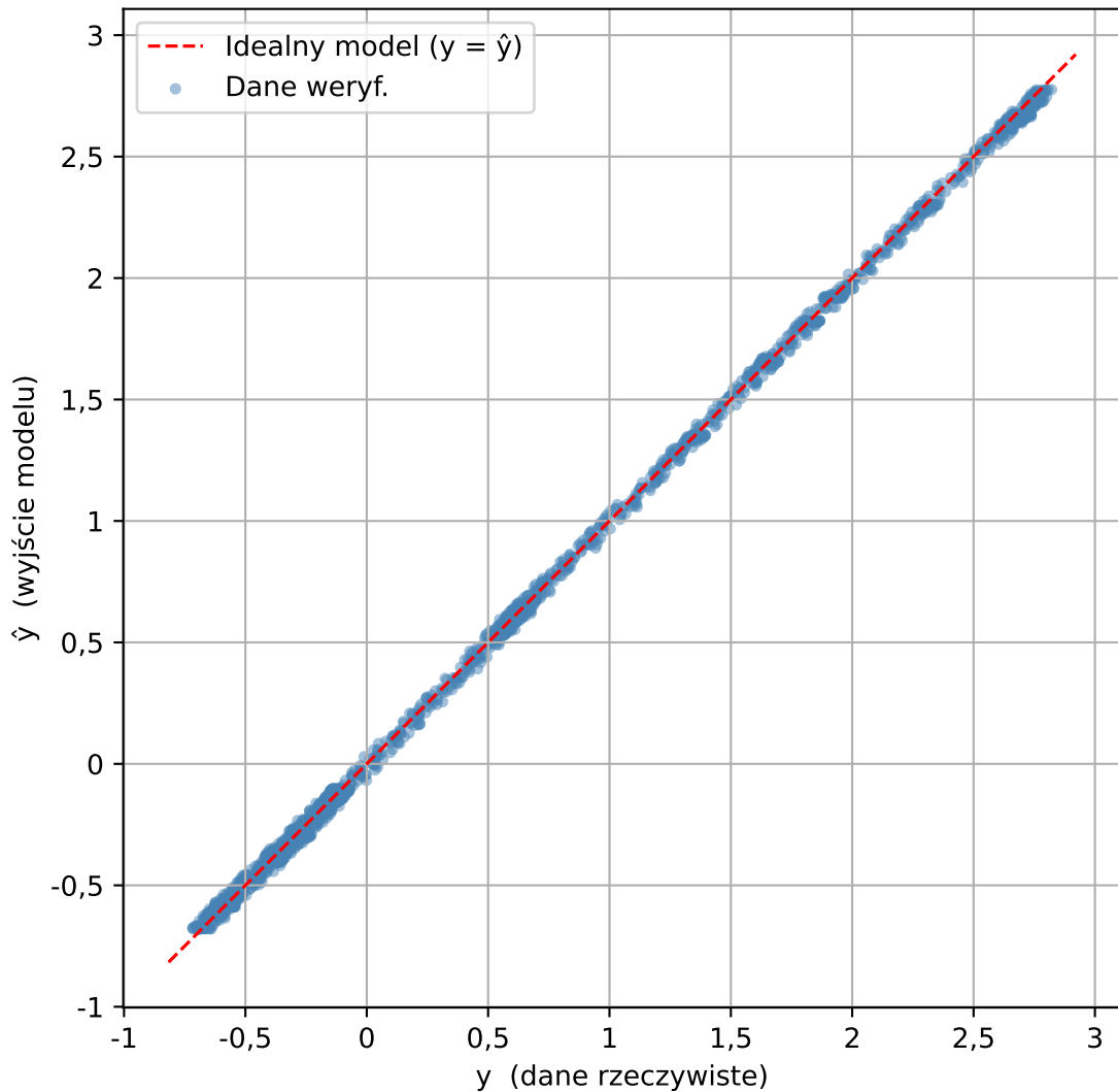
Relacja danych weryf. vs NARX(nA=14, deg=3) - z rekurencją
